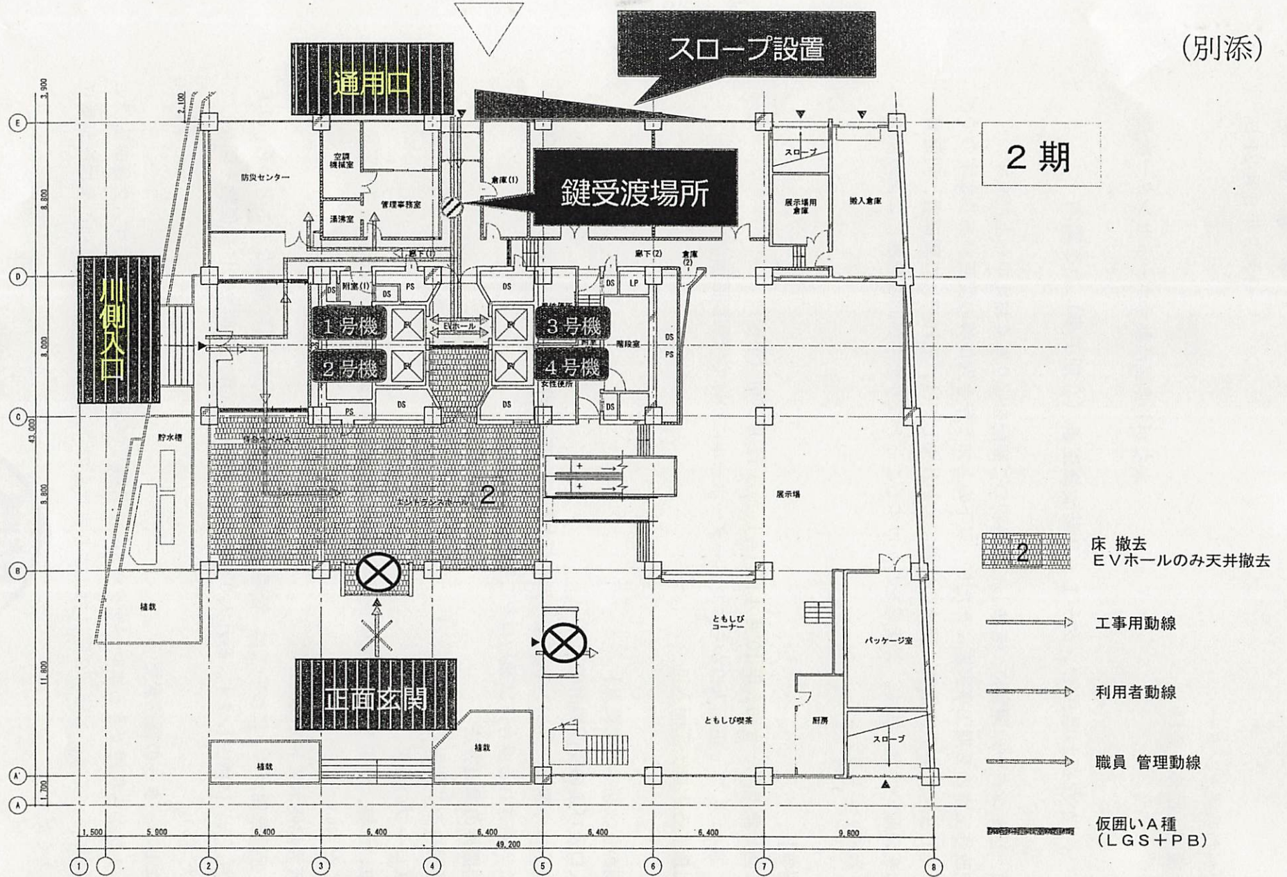
1階屋内仮設図(2) S=1:200
